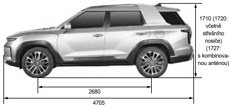
Boční pohled
