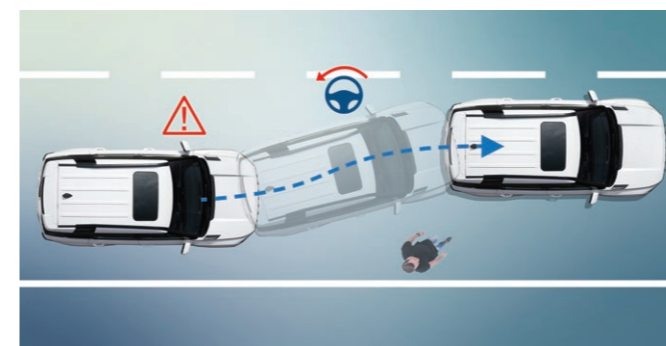
Systém udržování vozu v jízdním pruhu – automatické nouzové řízení Systém automaticky koriguje směr jízdy pro vyhnutí se překážce v jízdním pruhu.
